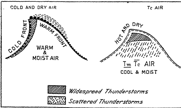
चित्र ५९—Tc और TmTc वायु राशियों के बीच अग्रभाग का बनना। विन्दी रेखा विक्षोभ के पहले अलगाव दर्शाती है।
